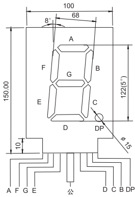
BL-SE500EA
